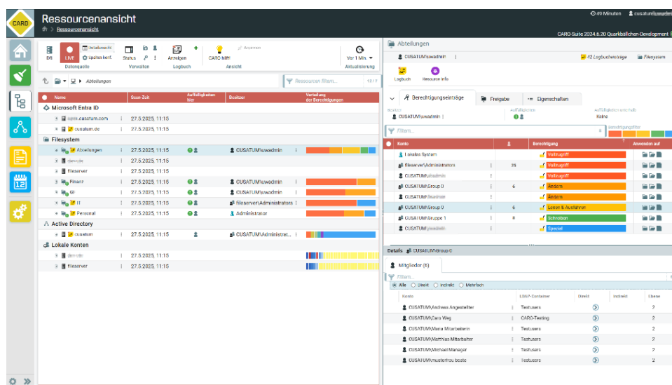
Live-Ansicht der Ist-Berechtigungen in der globalen Ressourcenansicht
