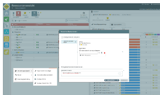
Verzeichnis-Besitzer ändern
